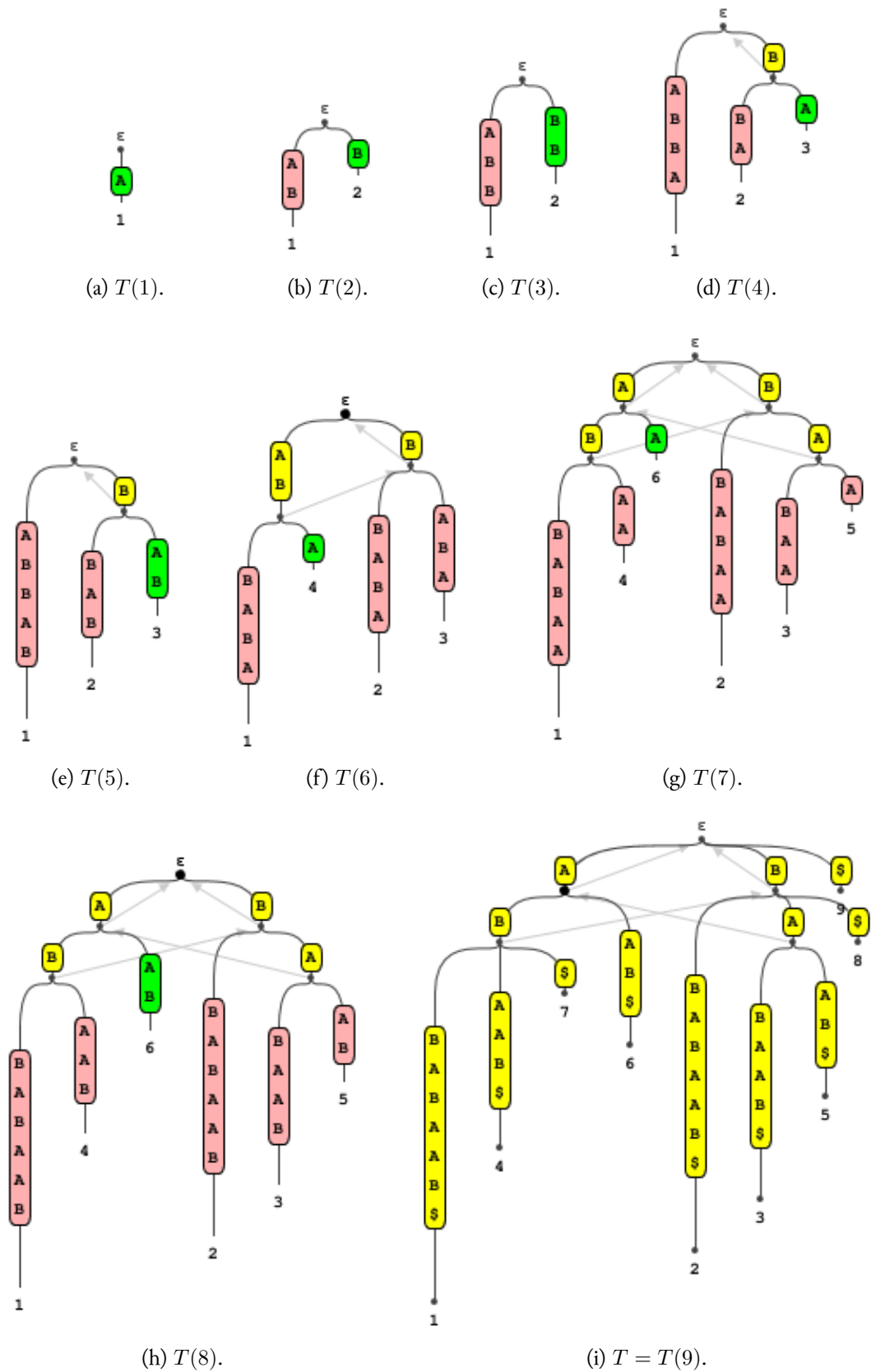
Obrázok 3.3: Sufixové stromy . Na obrázku sú sufixové stromy pre slová A, AB, ABB, ABBA, ABBAB, ABBABA, ABBABAA, ABBABAAB, ABBABAAB$. Šípky znázorňujú sufixové linky, ružovou a zelenou sú označené hrany, na ktoré sa bude v nasledujúcom, kroku aplikovať prvé pravidlo. Číslo označujú, na ktorom znaku začína daný sufix v slove.
