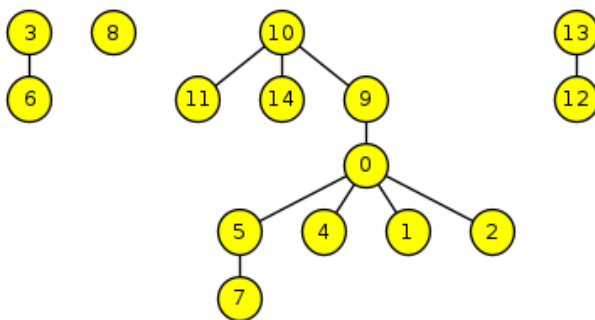
Obrázok 5.1: Vizualizácia union-find. Jednotlivé množiny sú vykresľované tesne a sú od seba oddelené pomyselnou zvislou čiarou.
