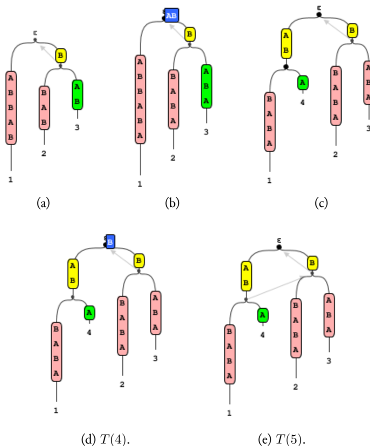
Obrázok 3.2: Rozšírenie stromu o písmenko A. (a) Suffixový strom pre slovo ABBAB. (b) Vykonali sme rozšírenie prvých prípadov – zvýšili sme index o jeden. Šli sme o hranu vyššie, zapamätali sme si, čo je na nej. Prešli sme po suffixovej linke a ideme hľadať zapamätaný reťazec. Keďže hľadáme z koreňa, zapamätaný reťazec nám nepomôže. Musíme nájsť celý reťazec w[4:5] . (c) Našli sme reťazec, nastal druhý prípad. Rozdelili sme hranu a vytvorili nový vrchol. Teraz musíme ísť po hrane vyššie, vyhľadať nové miesto pripojenia a vytvoriť suffixovú linku. (d) Našli sme miesto pripojenia a nastal tretí prípad: písmenko sa nachádza na niektorej z hrán. Vytvoríme suffixovú linku a skončíme. (e) Strom po rozšírení o písmenko A.
