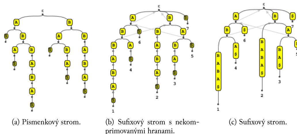
Obrázok 3.1: Rôzne typy suffixových stromov.
