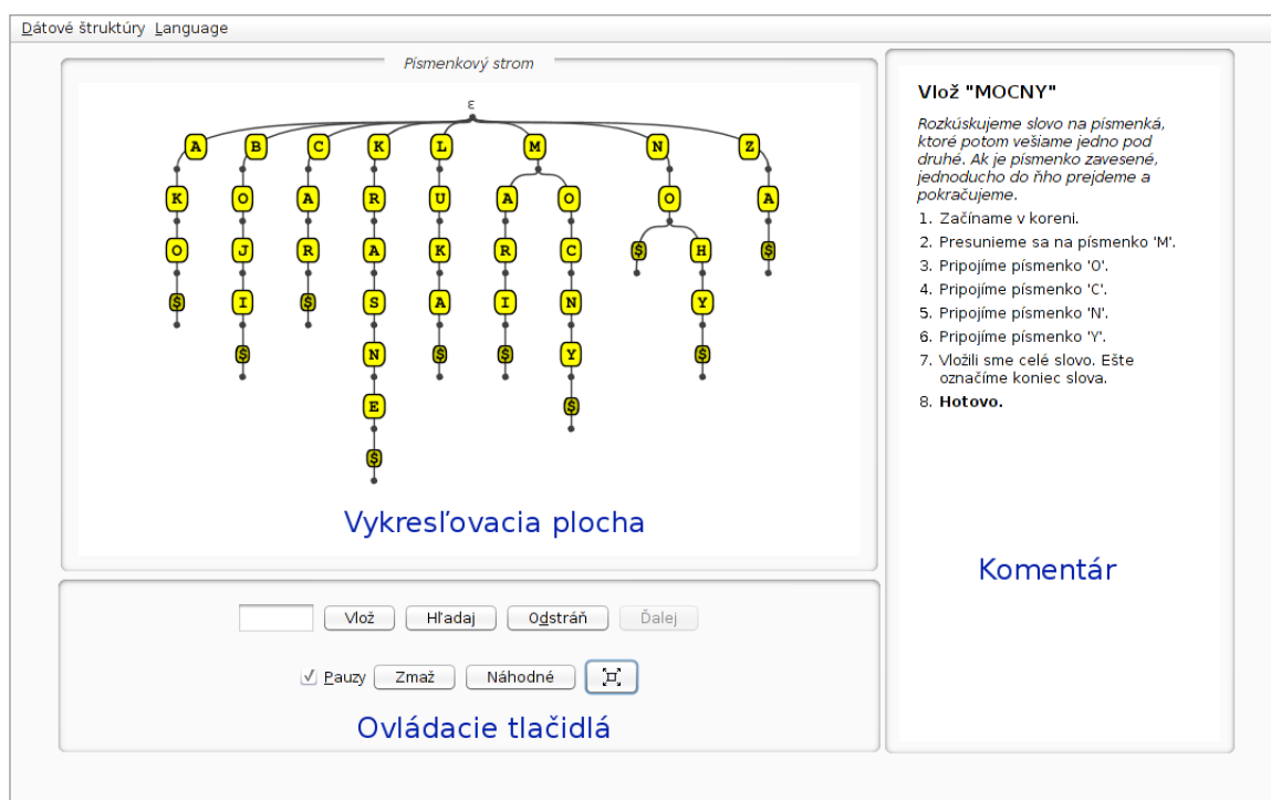
Obrázok 5.4: Grafické rozhranie softvéru Gnarley Trees . V hornej časti je lišta s menu pre výber dátových štruktúr a voľbu jazyka. Hlavnú časť obrazovky tvorí priestor na vykresľovanie dátových štruktúr. Vpravo je priestor na popis udalostí. Dole sú ovládacie tlačidlá.
