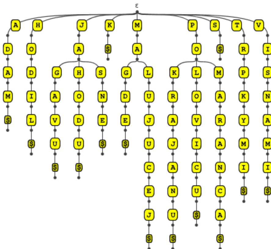
Obrázok 5.2: Vizualizácia písmenkového stromu. Písmenkový strom obsahuje slová ADAM$, HODIL$, JAGAVU$, JAHODU$, JASNE$, K$, MAGDE$, MALUJUCEJ$, POKRAJANU$, POLOVICU$, POMARANCA$, S$, TRPKYMI$, VYSNAMI$.
