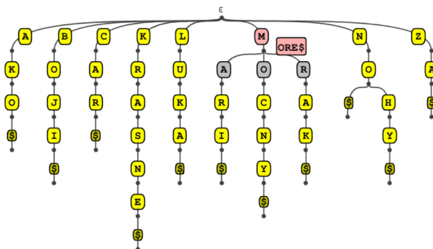
Obrázok 5.3: Hľadanie slova MORE$. Ružovou je vyznačené hľadané slovo. Šedou je označená množina písmen, na ktoré sa algoritmus práve pozerá.
