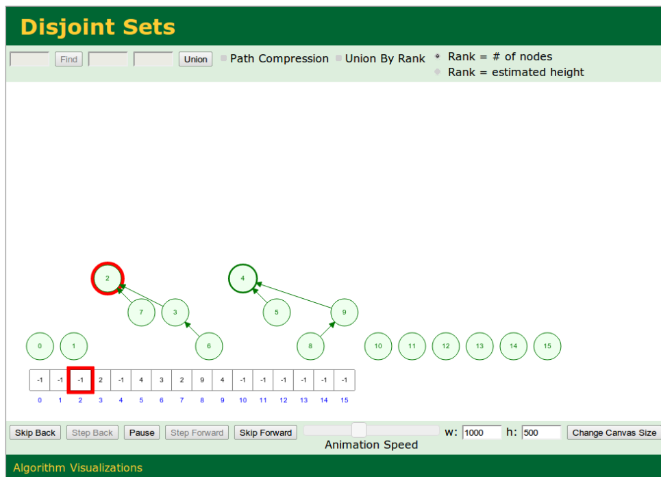
Obrázok 4.3: Softvér Data Structure Visualizations . Prebieha spájanie dvoch množín. Celá aplikácia beží v internetovom prehliadači.
